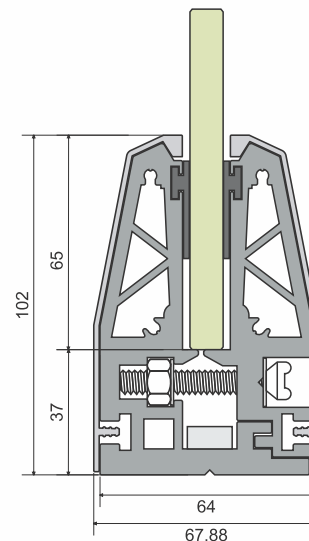
ALRL-01
